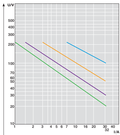
DC switching capacity E211 32A
