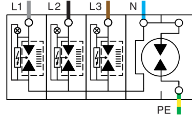
OVR T1+2 3N 15 255-7
