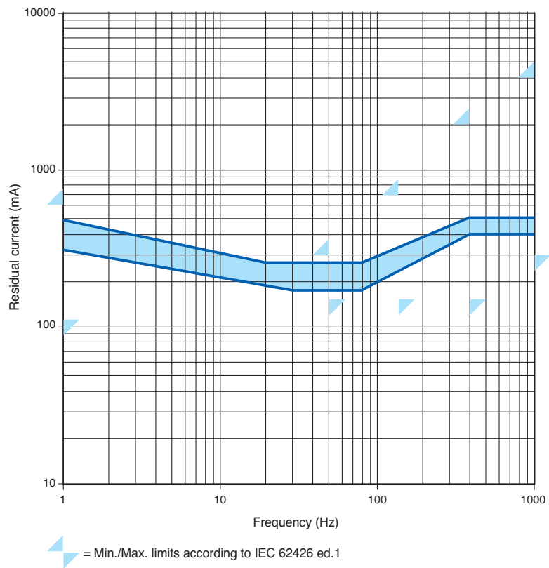
DDA 200 B type, 300 mA
