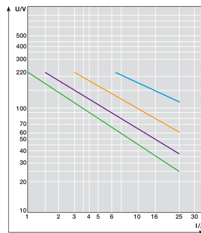
DC switching capacity E211 25A
